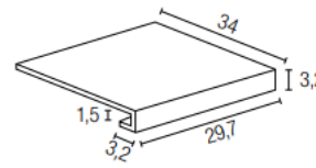
GRADONE A COSTA RETTA** 30x34 cm Rect NATURALE ± 9,5 mm
